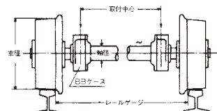
(B) 内メタルベアリング式
