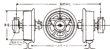
(A) 外メタルベアリング式 (標準型)
