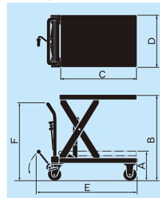
最高1,500(mm)まで 高揚程実現 TL-WH300-15 急降下防止バルブ付
